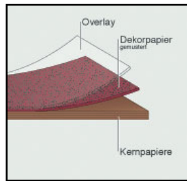
Abbildung: Typischer Aufbau einer Dekorativen Schichtstoffplatte
